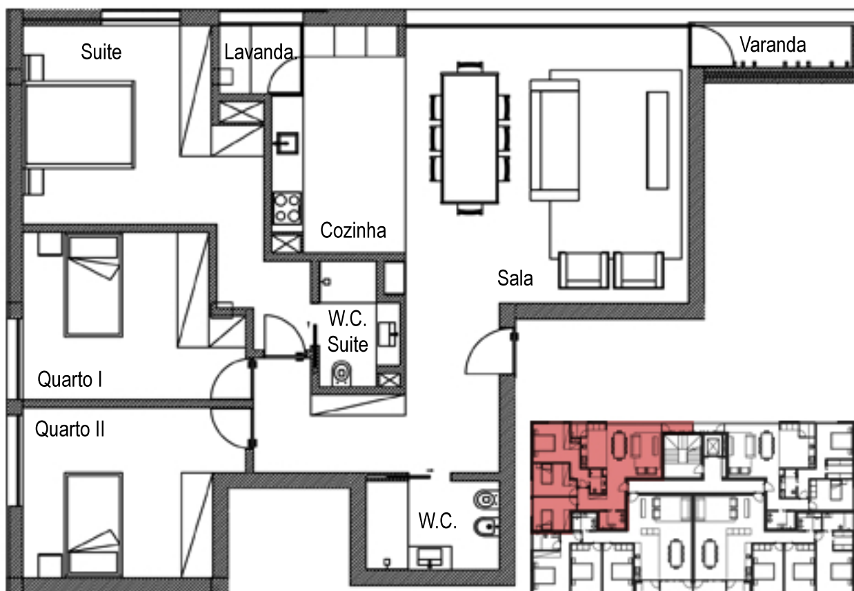
🕒 Planta Piso 2 Escala 1:50
