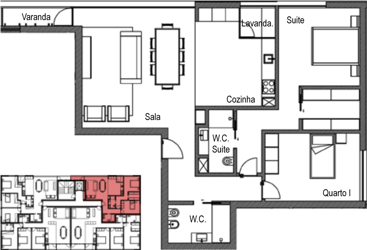
⌚ Planta Piso 2 Escala 1:50
