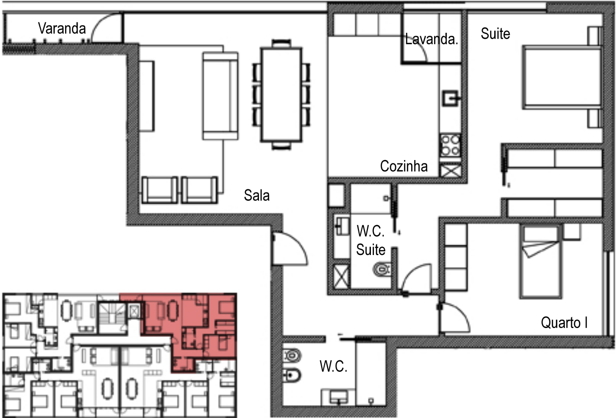
⌚ Planta Piso 1 Escala 1:50
