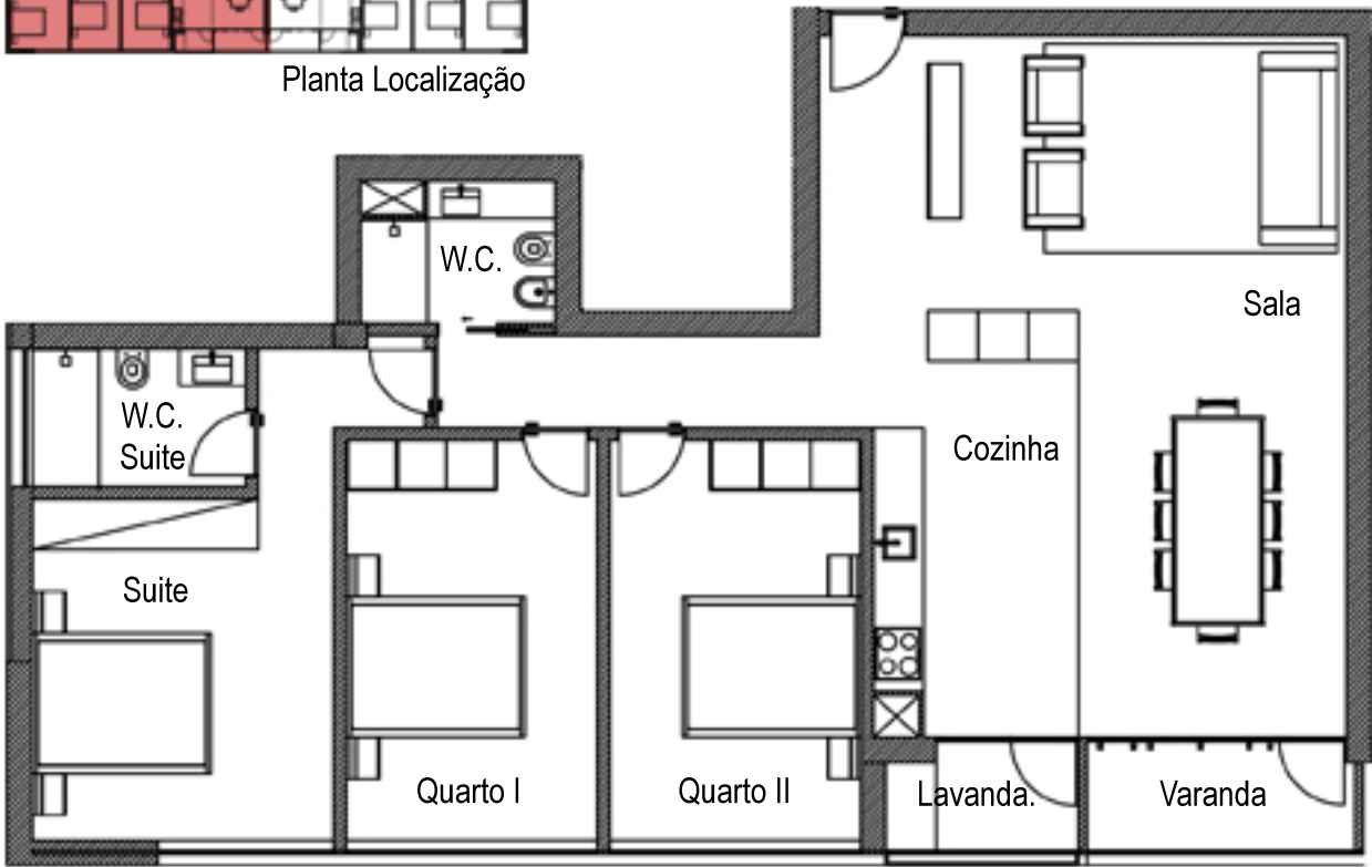
⌚ Planta Piso 2 Escala 1:50
