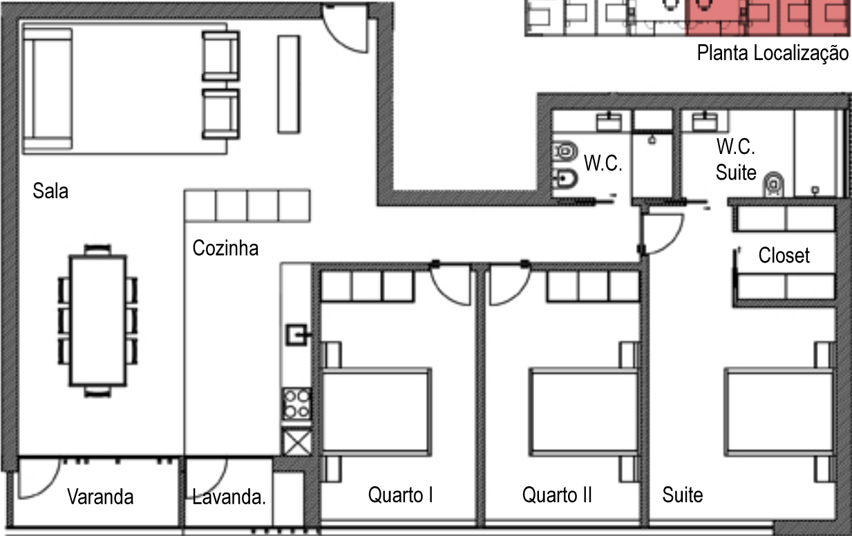
⌚ Planta Piso 3 Escala 1:50
