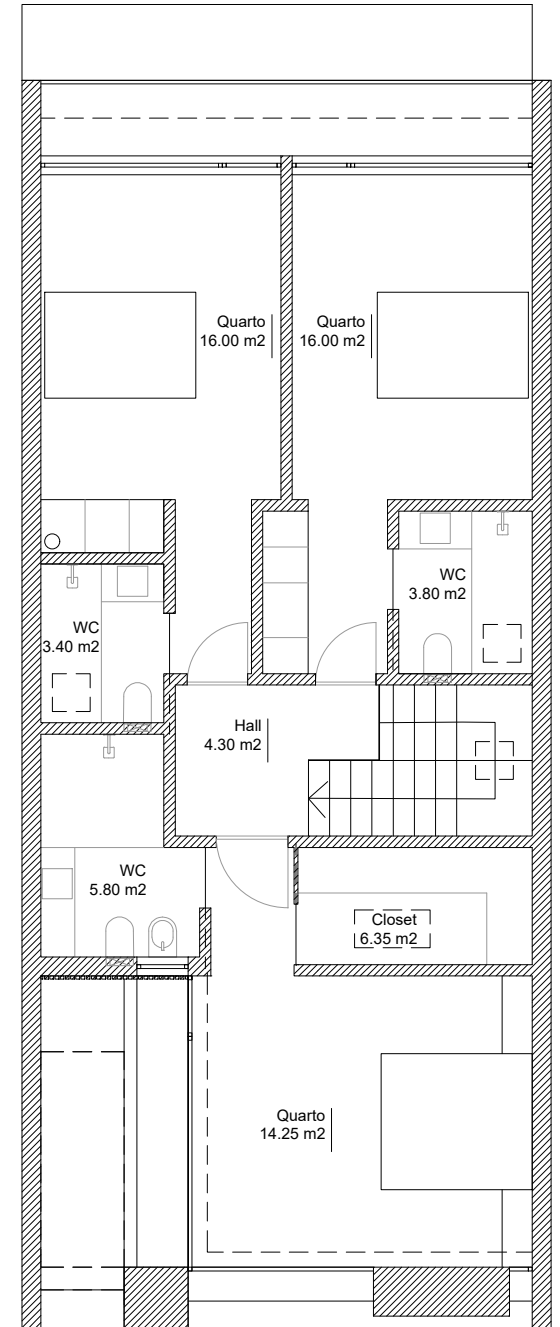
PISO 1
