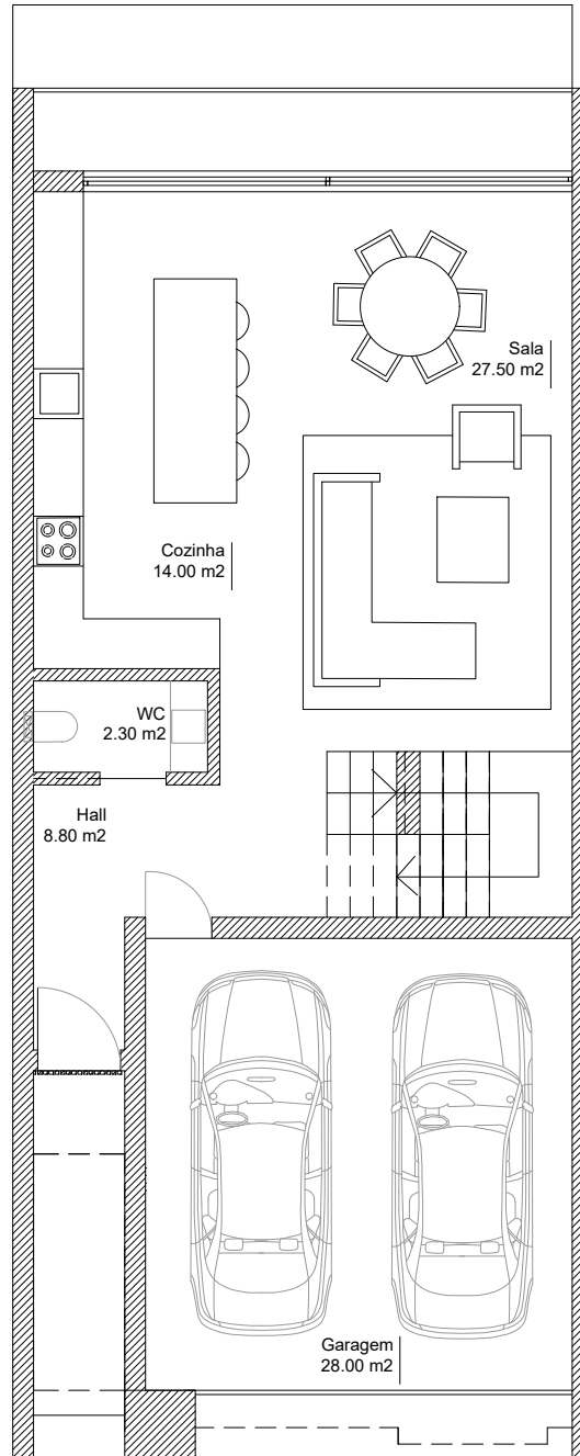
PISO 0
